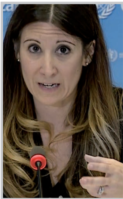
كيرخوف
