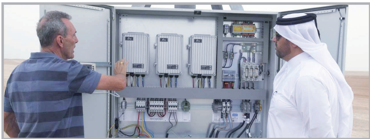
■ نظم الري المحوري لحصاد تعمل بالطاقة الشمسية
